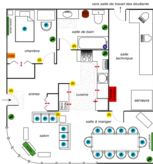
Laboratoire DOMUS - Département d'Informatique - Université de Sherbrooke plan d'aménagement de la partie Habitat et salle technique
